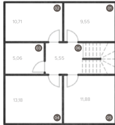
EBENE -01
