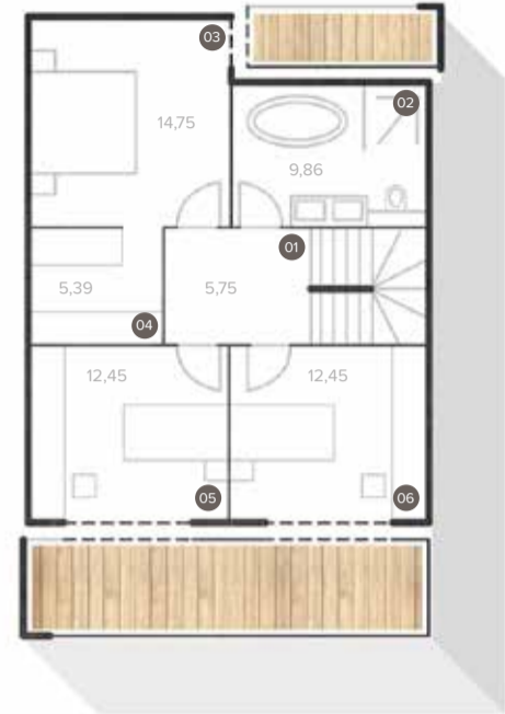
EBENE 01
